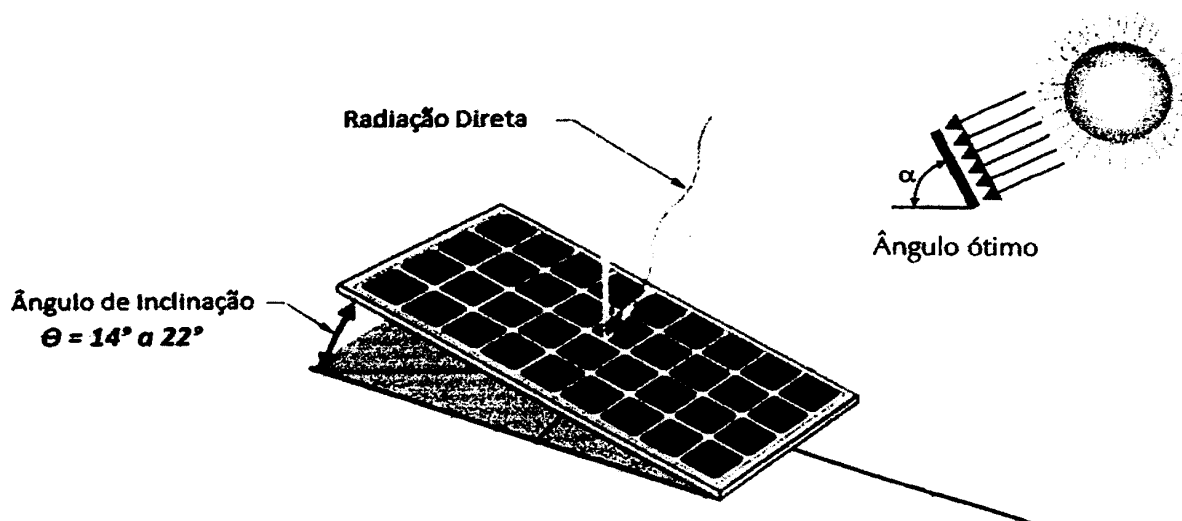
Imagem 01: Posição ideal do módulo fotovoltaico
